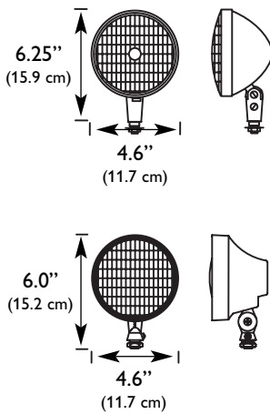
Metal Chrome & Thermoplastic Sealed Beam Par 36
